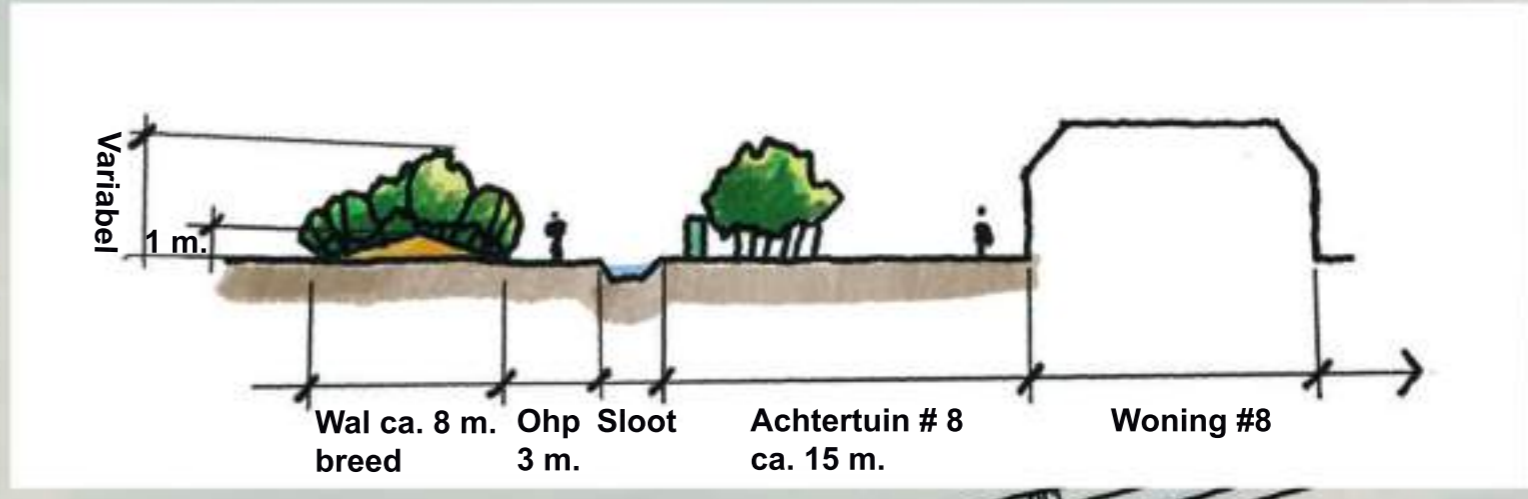
Principe aardenwal met dichte beplanting als geluidsbuffer
